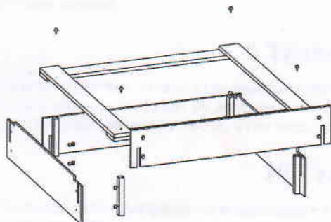
Рис.2 Схема сборки
