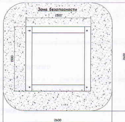
Рис.3 Основные размеры, схема расположения фундаментов и зона безопасности
